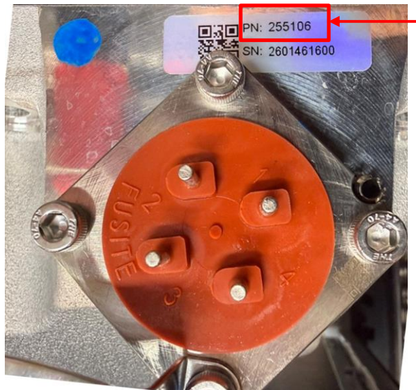
图 2 - IGV 喉管外壳零件号位置
