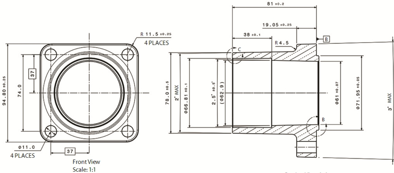
Section View A-A Scale: 1:1
